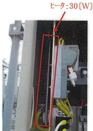
赤相ヒータ外観 ○KSW「切」位置が湿度センサによる自動運転 ○200[V]、30[W]、70[%]自動運転(74%で入、66%で切)
