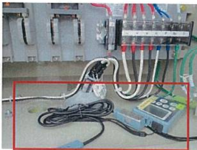
赤相内の部温・湿度測定状況 (□が温・湿度計)
